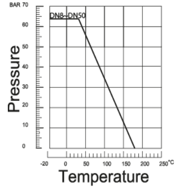
pressure - temperature druk - temperatuur
